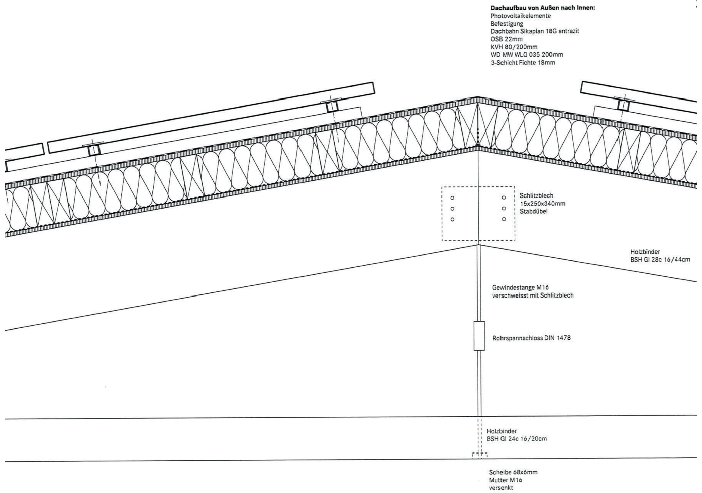
Schnitt Dach
